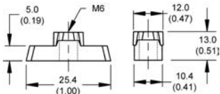
导轨螺母 产品型号 BMS-RN-1/4-20
