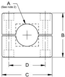
夹具 产品型号 BMS-B-xx
